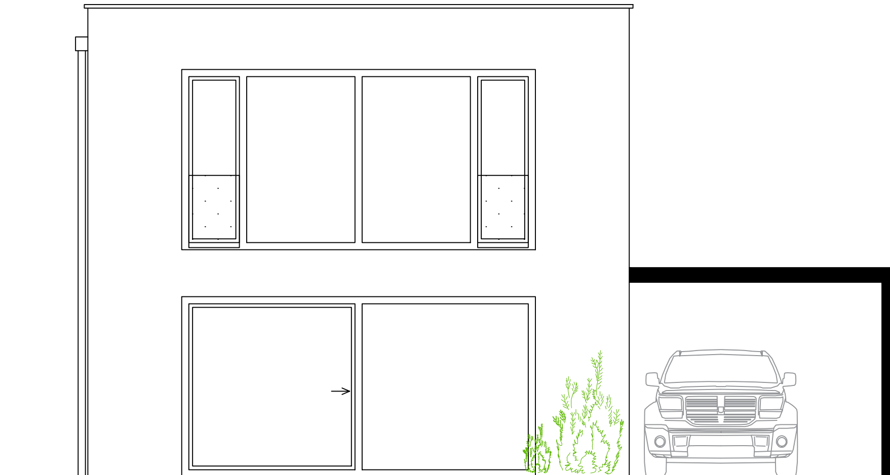
Zadný pohľad
